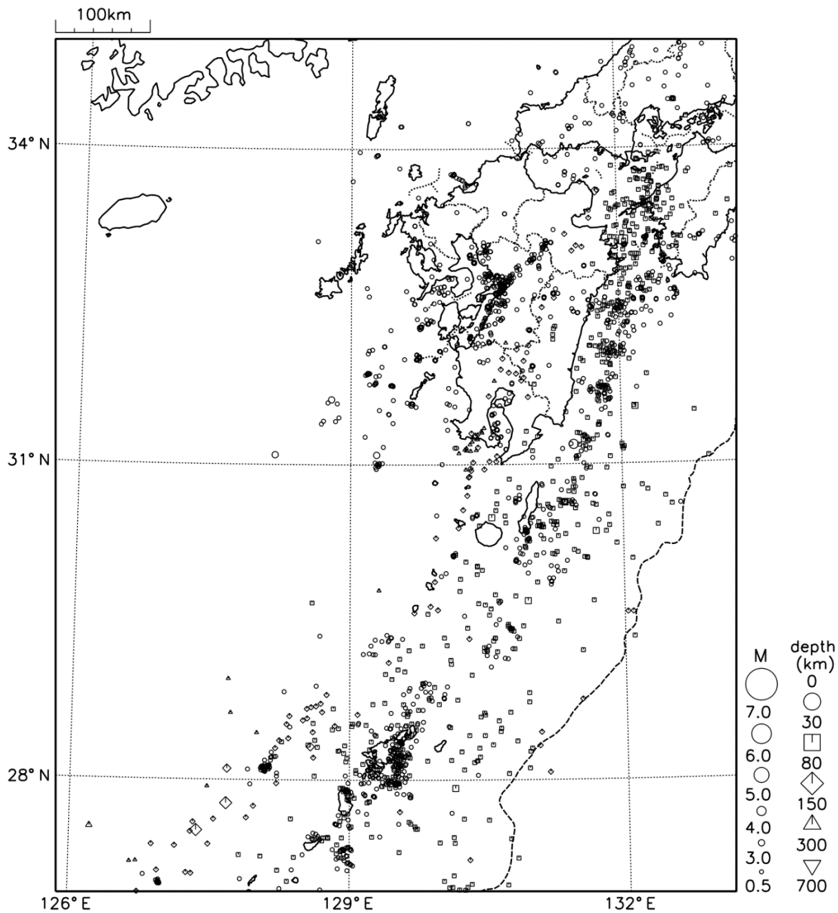
図9 九州地方の震央分布図（2021年9月1日～9月30日、 M \geq 0.5 ）
