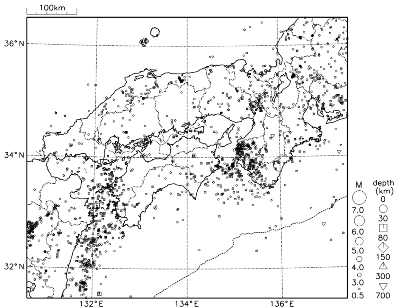
図8 近畿・中国・四国地方の震央分布図（2021年9月1日～9月30日、 M \geq 0.5 ）
