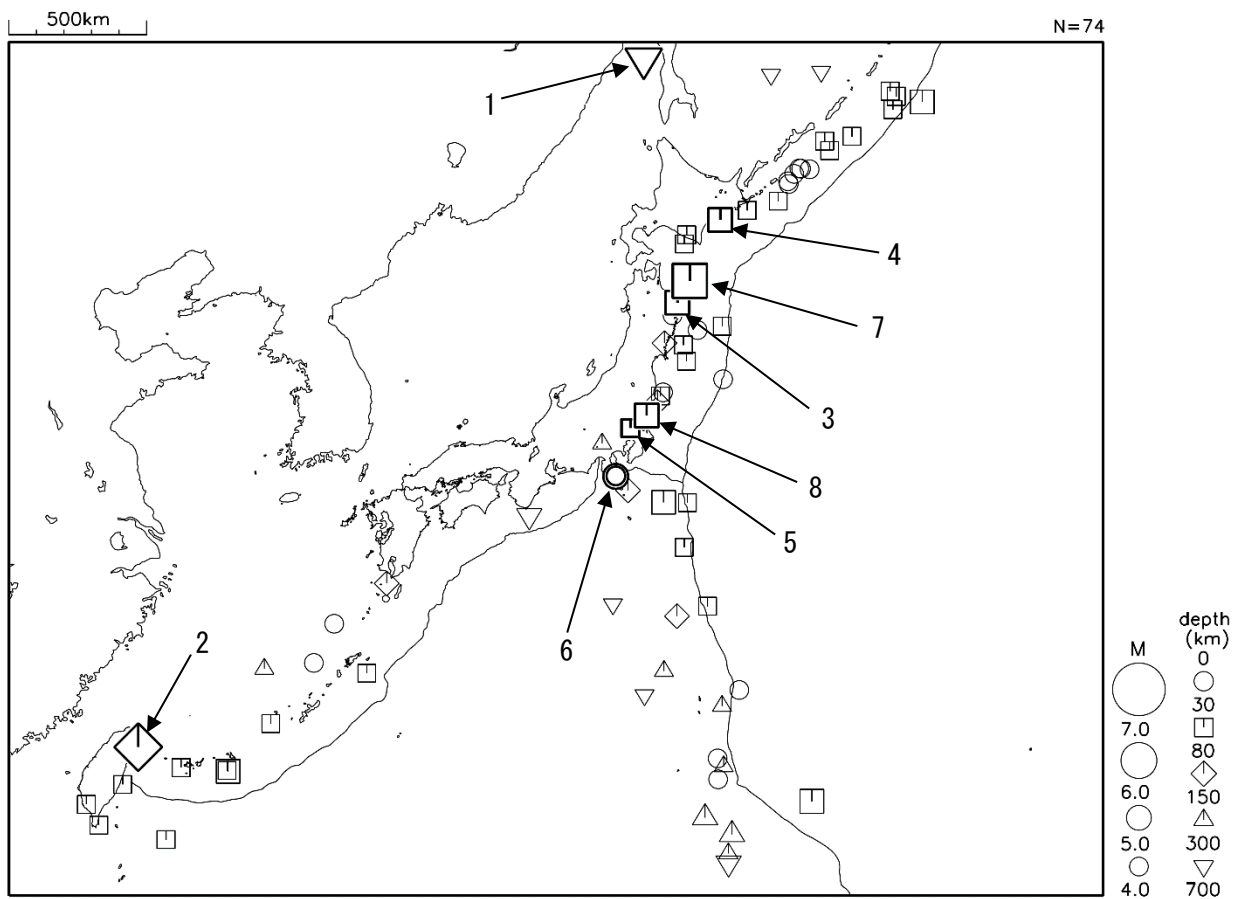
図3 令和2年12月に発生したM4.0以上の地震（図中の番号は、表の番号に対応）
