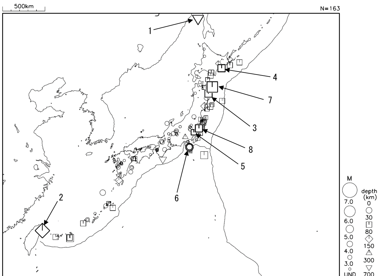
図2 令和2年12月に震度1以上を観測した地震（図中の番号は、表の番号に対応）
