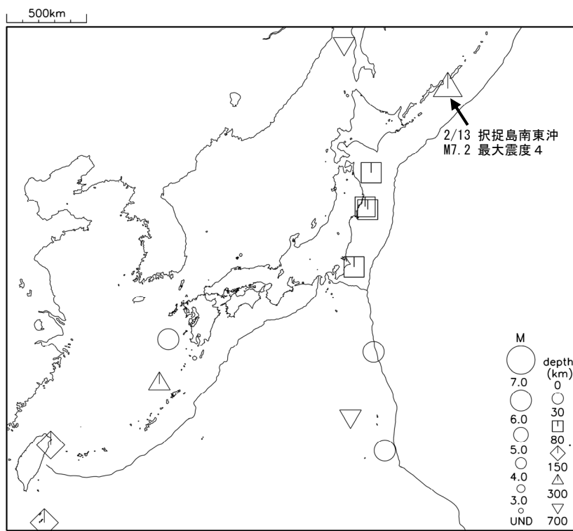
図2 2020年に発生した M6.0以上の地震の震央分布図 2020年中で最大規模の地震に矢印をつけた
