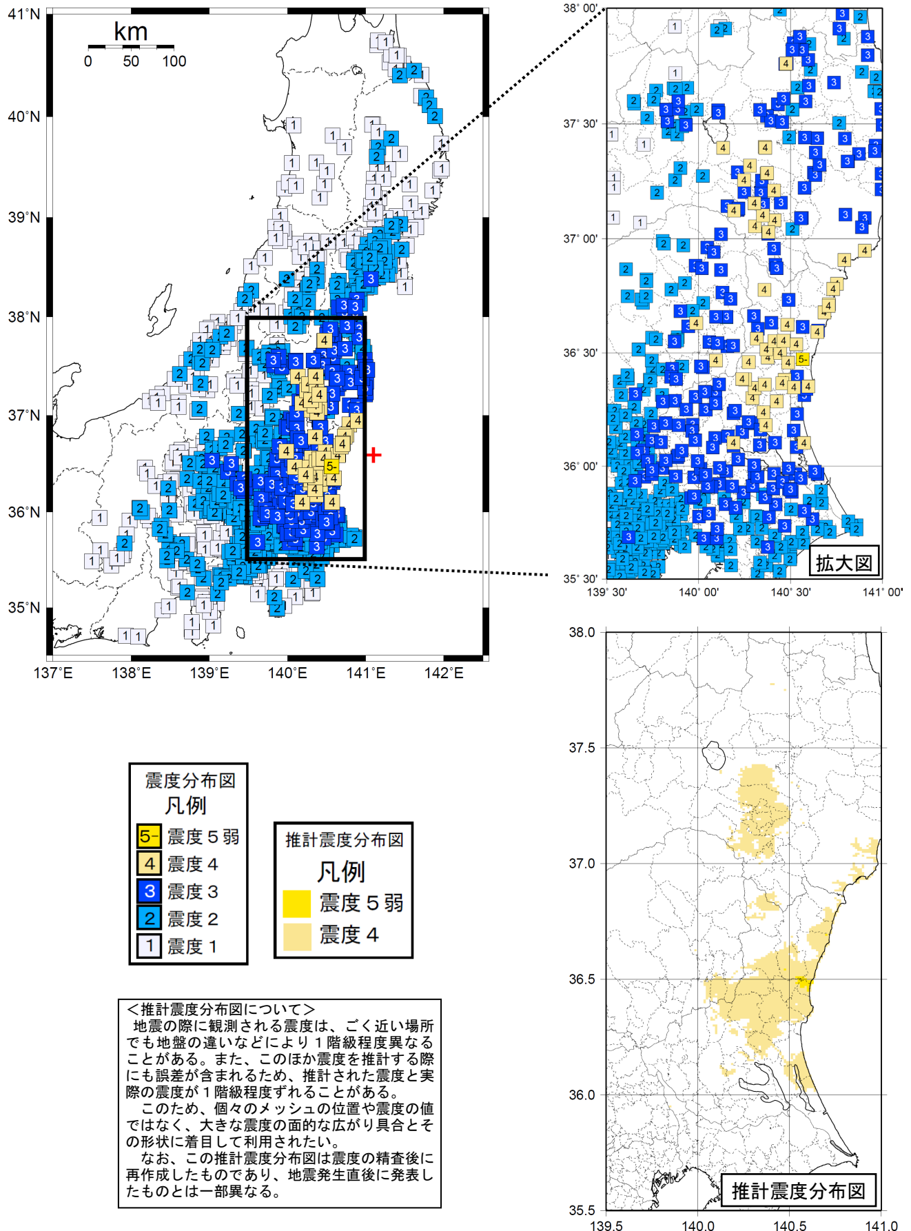
図4 震度分布図
