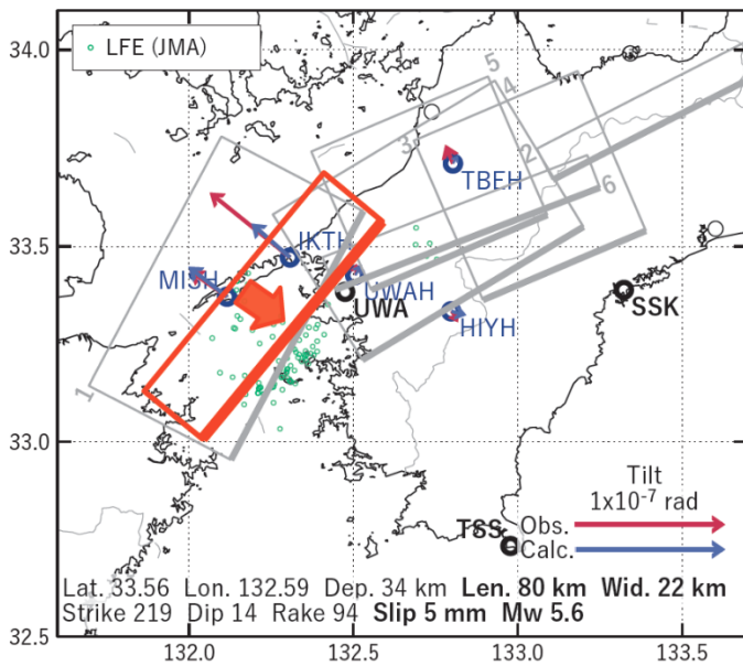
図6 2020/05/17-20AMの歪・傾斜変化（図5[A]）を説明する断層モデル。
