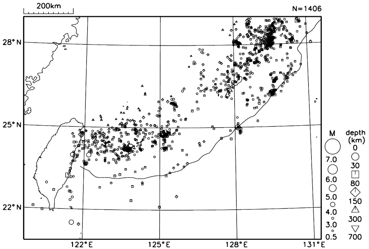
図10 沖縄地方の震央分布図（2019年5月1日～5月31日、 M \geq 0.5 ）
