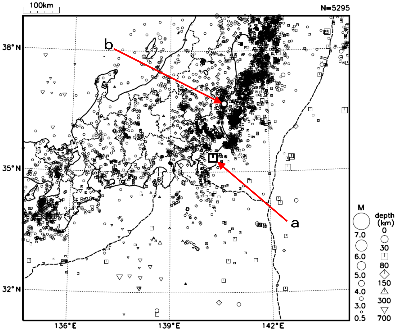
図7 関東・中部地方の震央分布図（2019年5月1日～5月31日、 M \geq 0.5 ）
