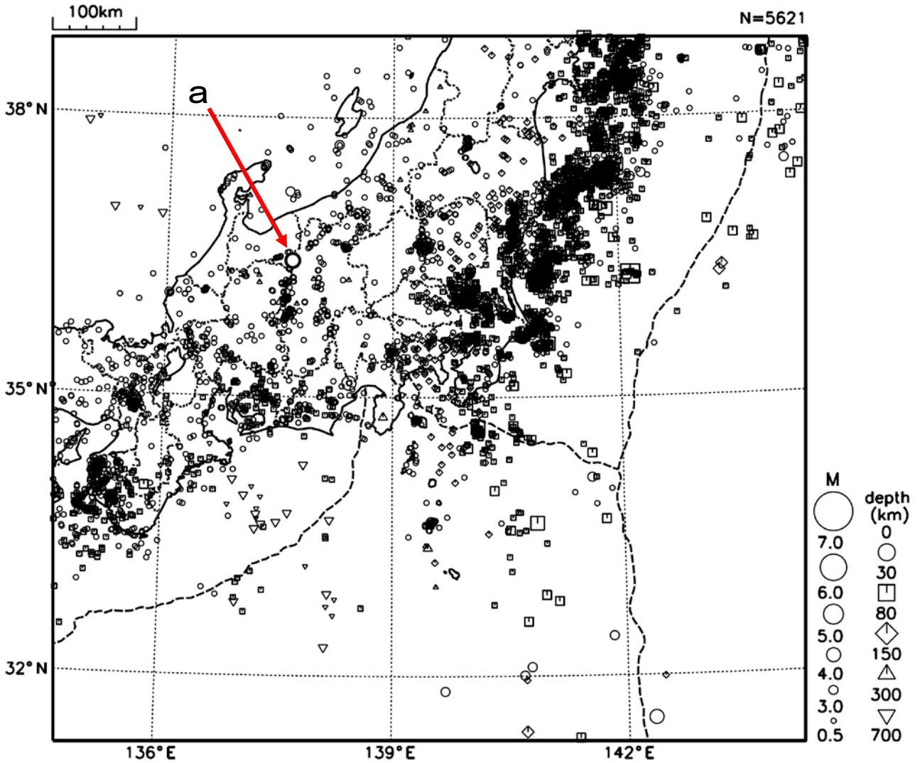
図7 関東・中部地方の震央分布図 (2019年2月1日～2月28日、 M \geq 0.5 )
