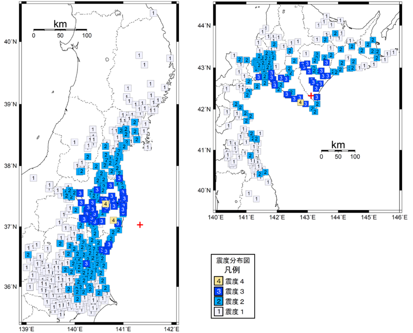
図4 震度分布図
