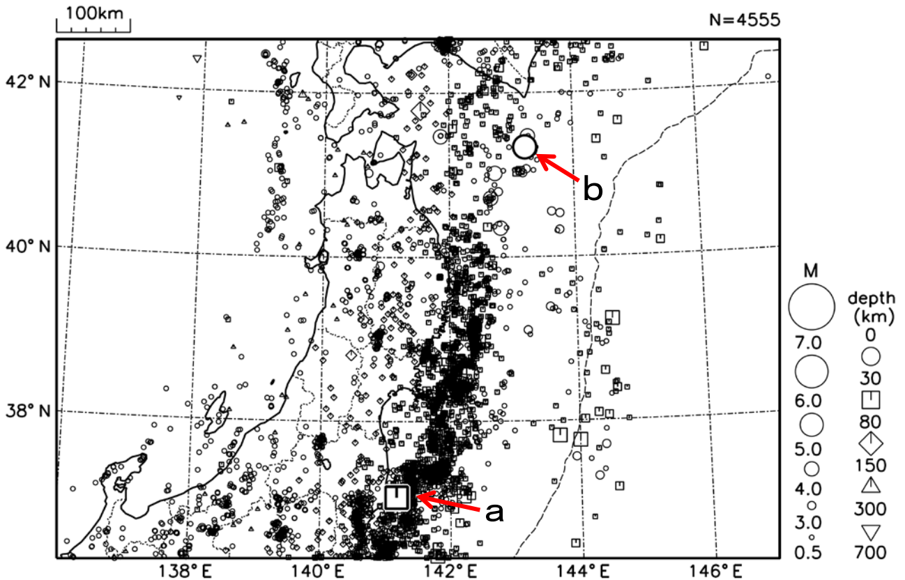
図6 東北地方の震央分布図 (2018年11月1日~11月30日、 M \geq 0.5 )
