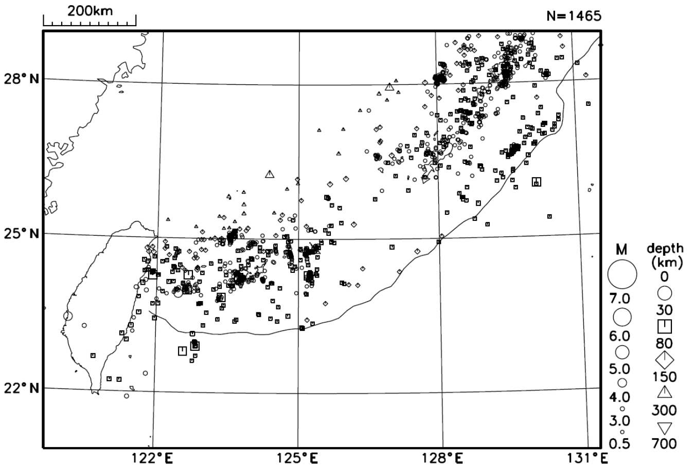
図10 沖縄地方の震央分布図(2018年11月1日~11月30日、M \geq 0.5)
