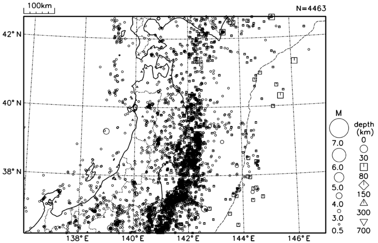
図6 東北地方の震央分布図 (2018年6月1日～6月30日、 M \geq 0.5 )
