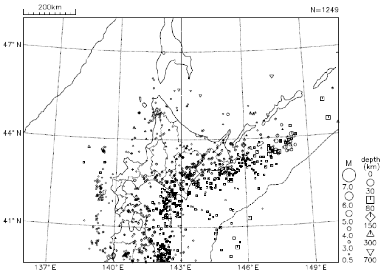
図5 北海道地方の震央分布図（2018年6月1日～6月30日、 M \geq 0.5 ）
