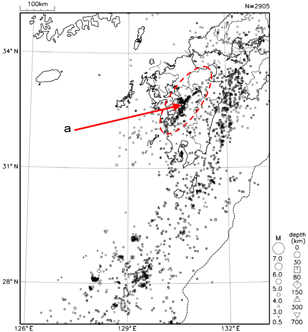
図9 九州地方の震央分布図 (2018年5月1日～5月31日、 M \geq 0.5 )
