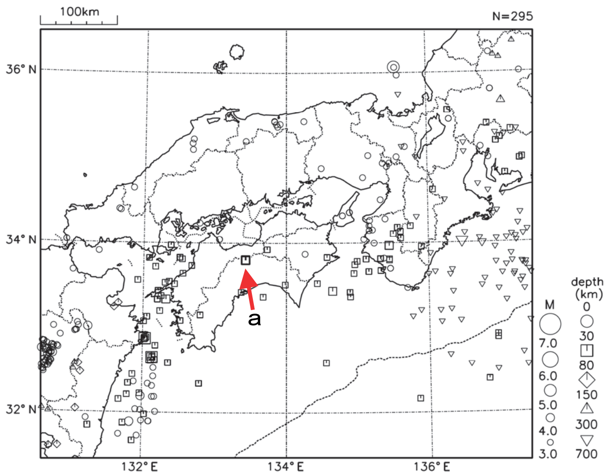
図 8 近畿・中国・四国地方の震央分布図（2017 年 1 月 1 日～12 月 31 日、 M \geq 3.0 ）
