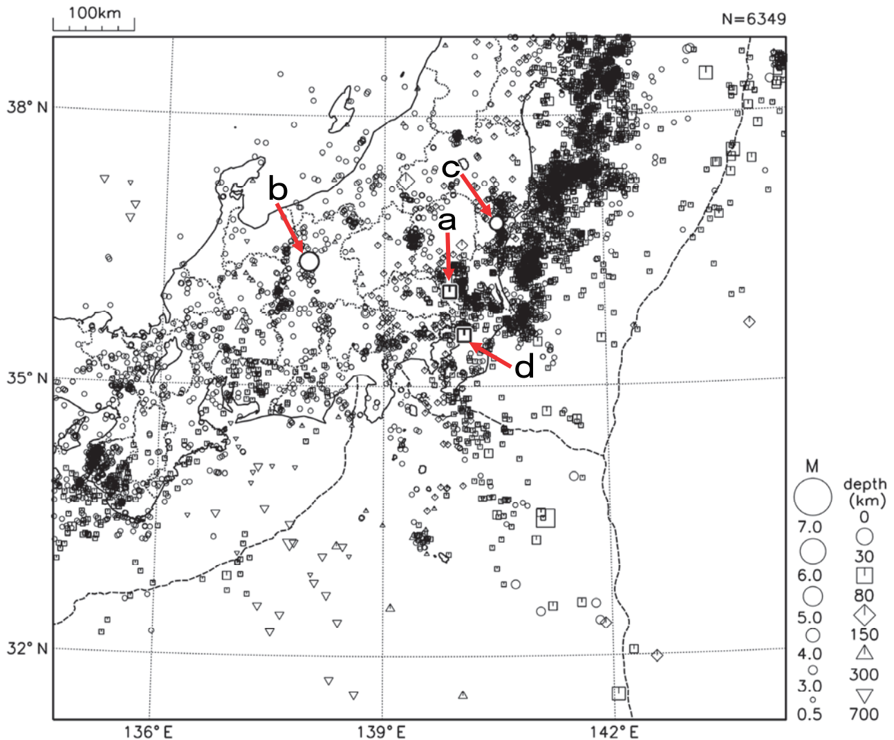
図6 関東・中部地方の震央分布図（2017年12月1日～12月31日、M \geq 0.5）
