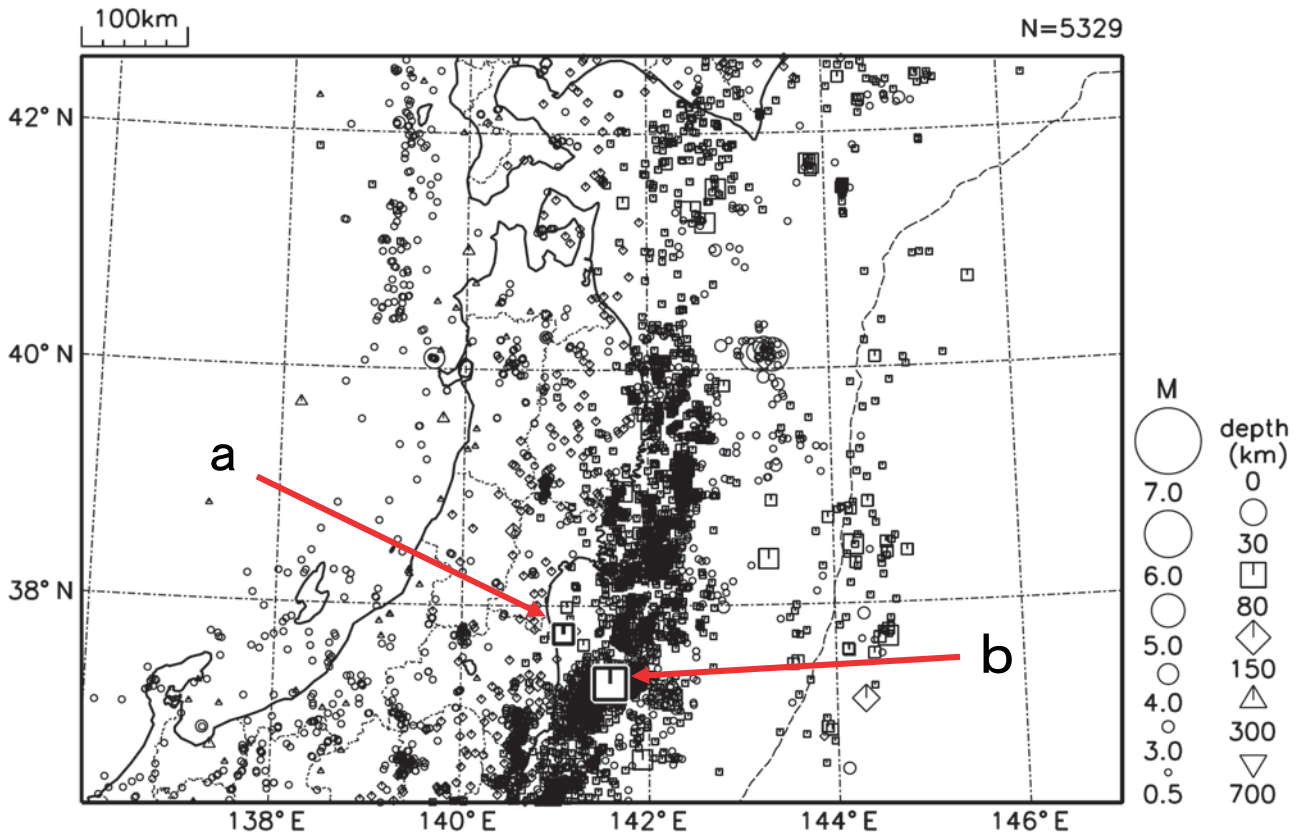
図5 東北地方の震央分布図（2017年7月1日～7月31日、 M \geq 0.5 ）
