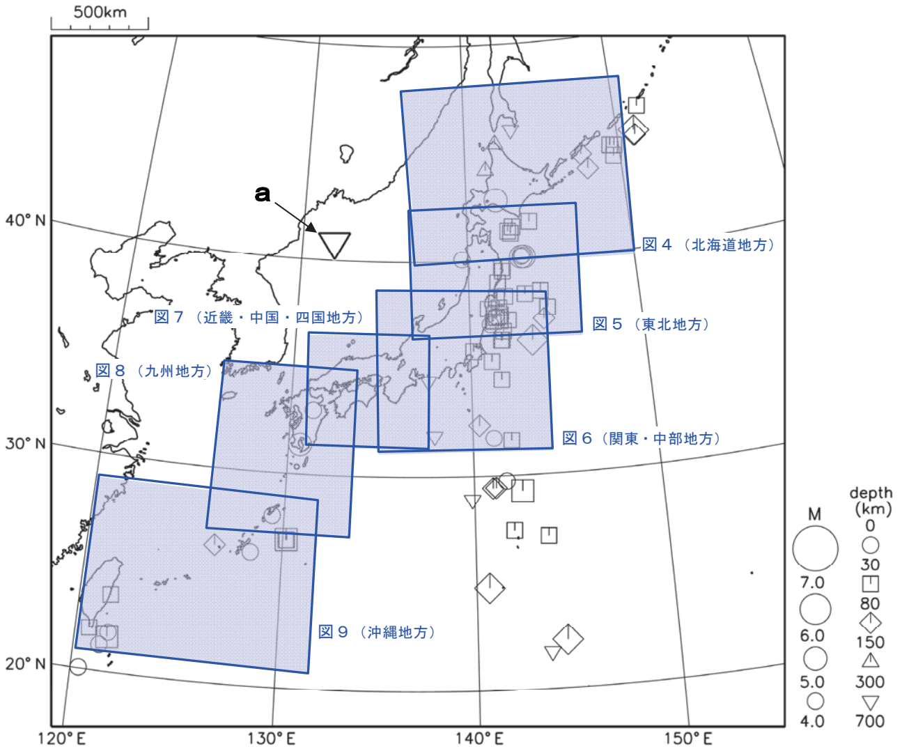
図 10 日本周辺で発生した主な地震の震央分布図（2017 年 7 月 1 日～7 月 31 日、 M \geq 4.0 ）
