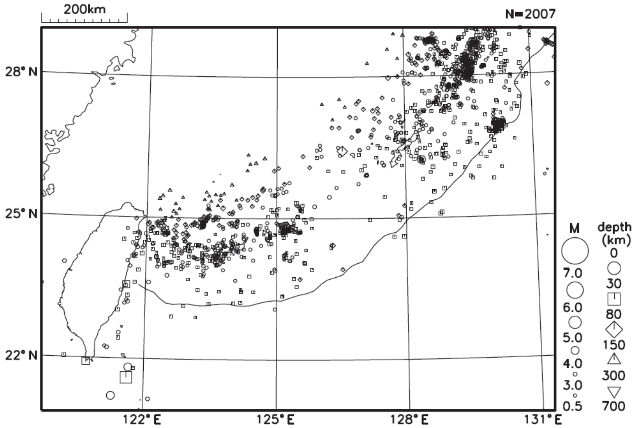
図9 沖縄地方の震央分布図（2017年7月1日～7月31日、 M \geq 0.5 ）
