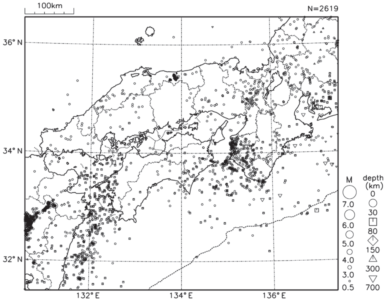
図7 近畿・中国・四国地方の震央分布図（2017年7月1日～7月31日、 M \geq 0.5 ）
