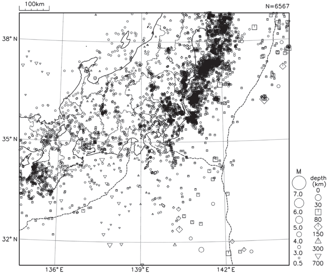
図6 関東・中部地方の震央分布図（2017年7月1日～7月31日、 M \geq 0.5 ）
