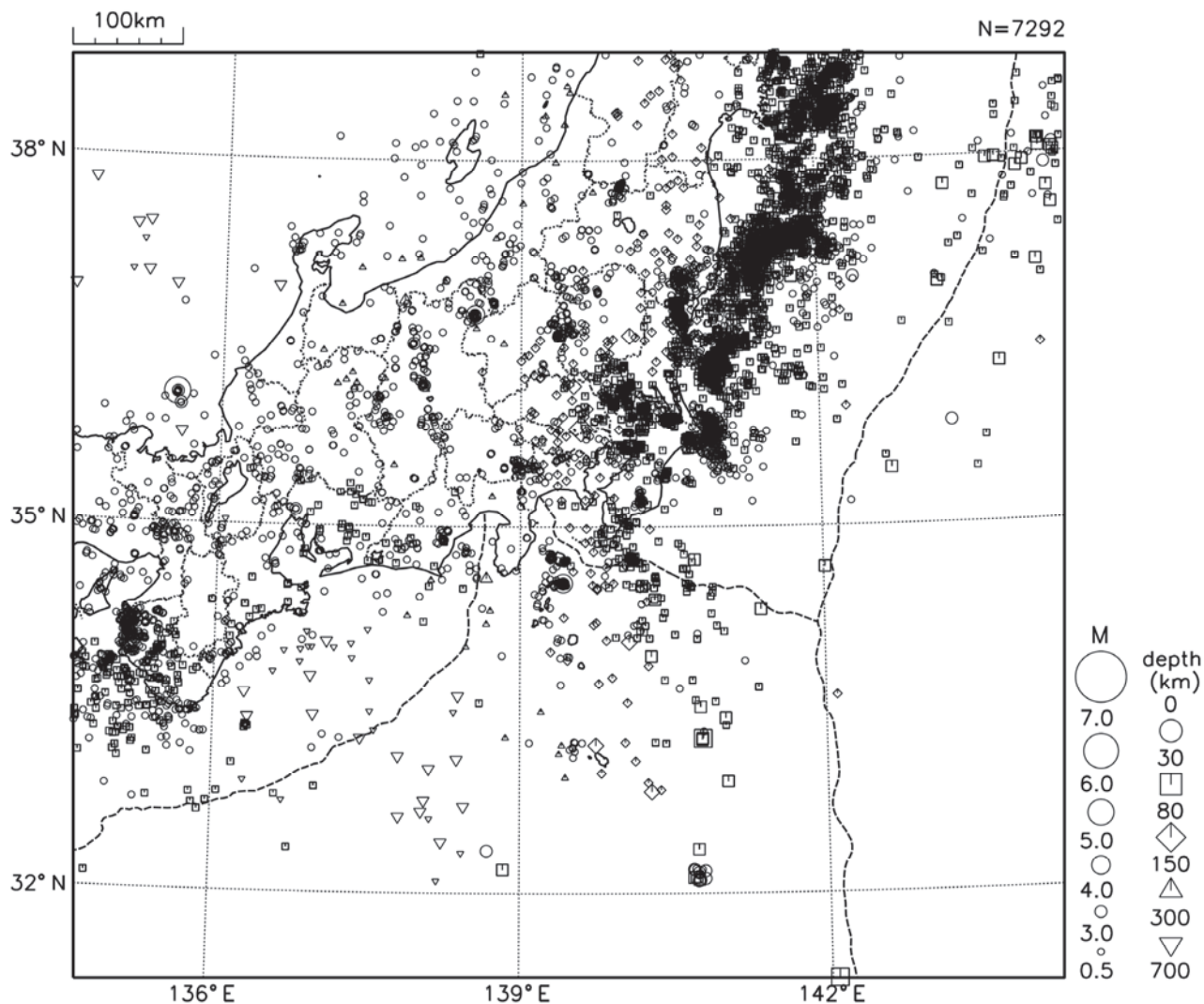
図6 関東・中部地方の震央分布図（2017年5月1日～5月31日、 M \geq 0.5 ）
