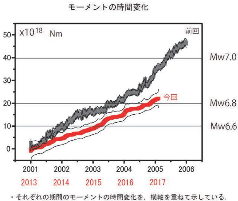
図 16 国土地理院 GNSS 観測結果による、長期的ゆっくりすべりの発生を示唆する非定常地殻変動から推定される累積すべり分布及びモーメントの時間変化の比較
