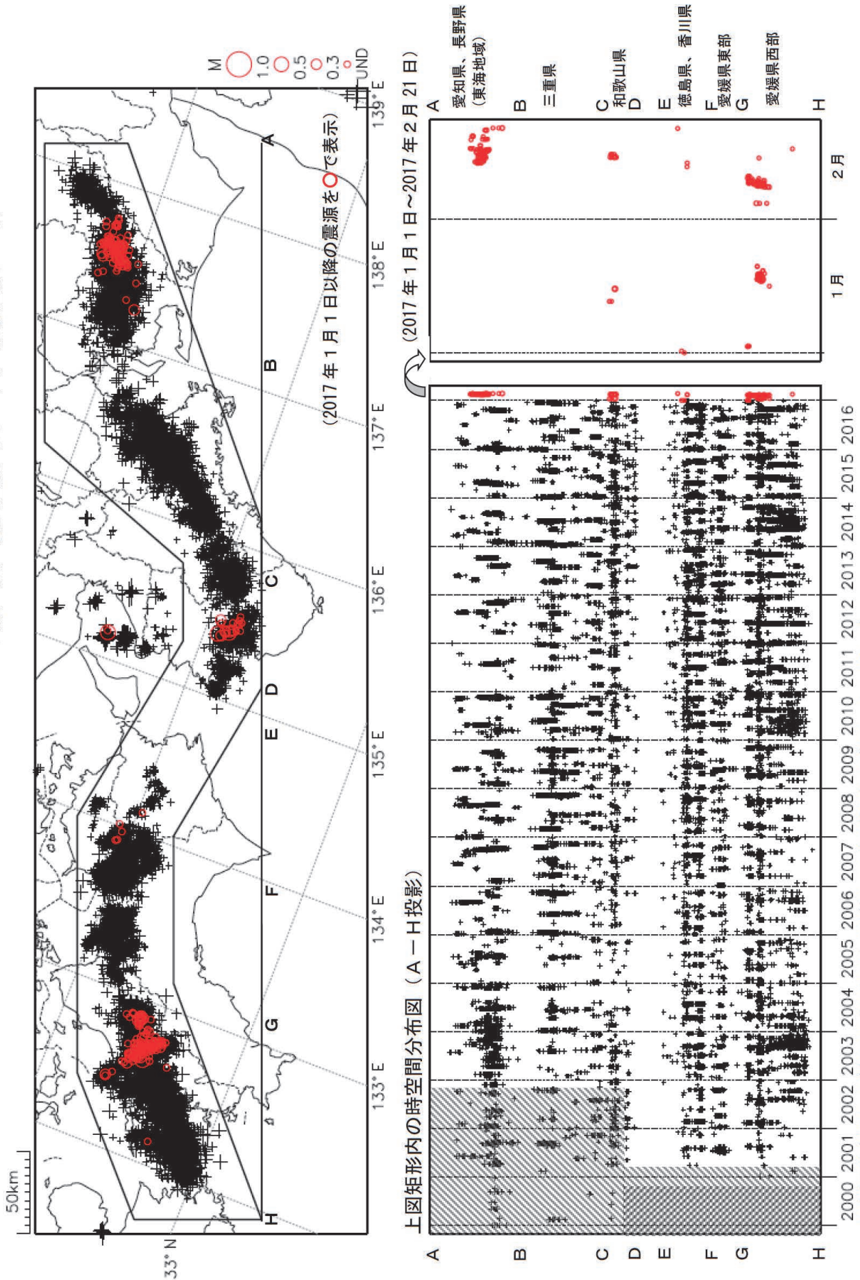
図 4 深部低周波地震活動（2000 年 1 月 1 日～2017 年 2 月 21 日）
