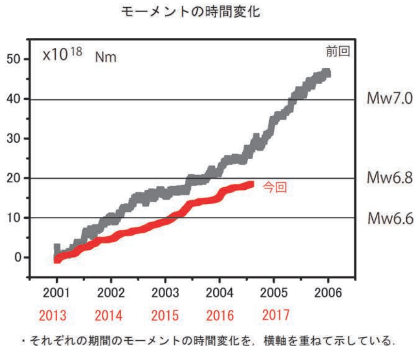
図 16 国土地理院 GNSS 観測結果による、長期的ゆっくりすべりの発生を示唆する 非定常地殻変動から推定される累積すべり分布及びモーメントの時間変化の比較
