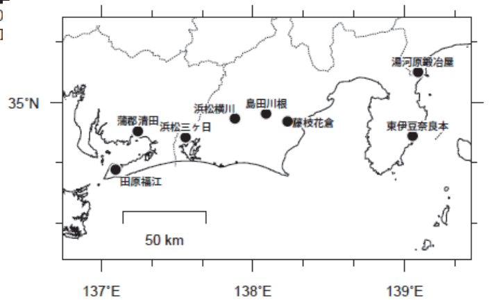
図 3-2 体積ひずみ計の配置図
