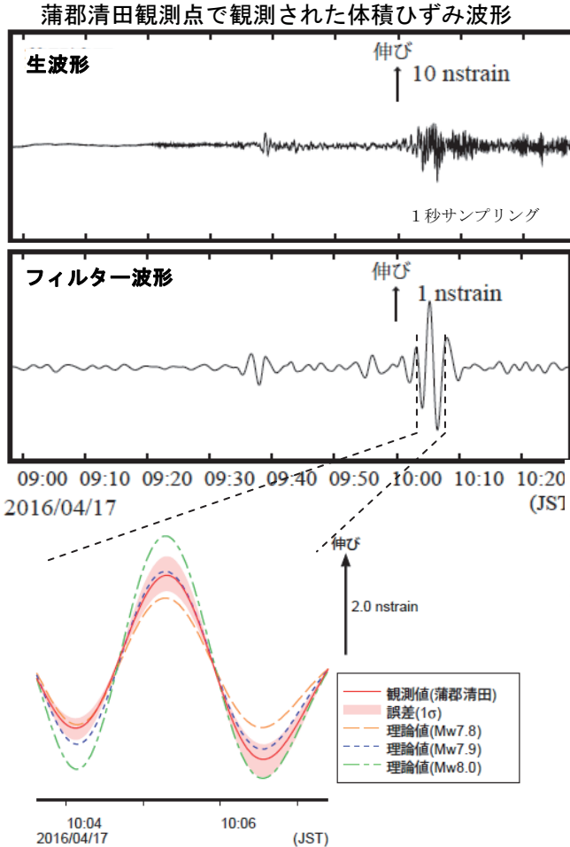
図 3-1 蒲郡清田観測点の観測波形と理論波形の振幅比較 データには周期 120-333 秒のバンドパスフィルタを時間軸の正逆両方向にかけている。網掛けは誤差 (1σ) の範囲を示す。
