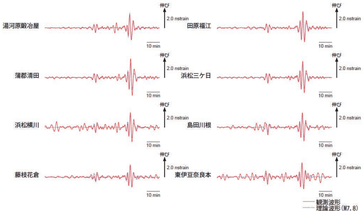
図 3-3 理論波形と体積ひずみ観測点 8 ヲ所の観測波形との比較 データには周期 120-333 秒のバンドパスフィルタを時間軸の正逆両方向にかけている。
