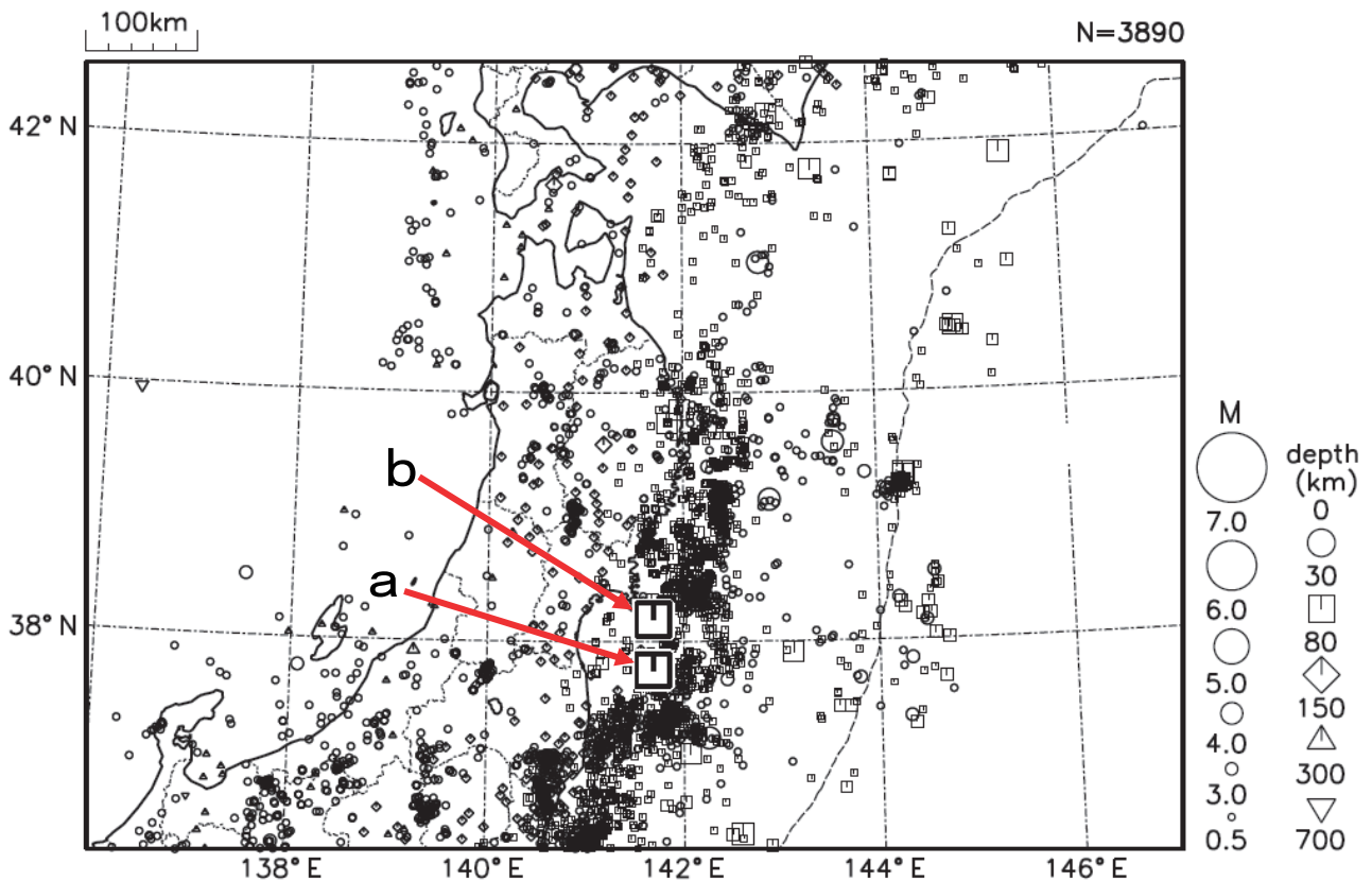
図5 東北地方の震央分布図（2016年4月1日～4月30日、 M \geq 0.5 ）
