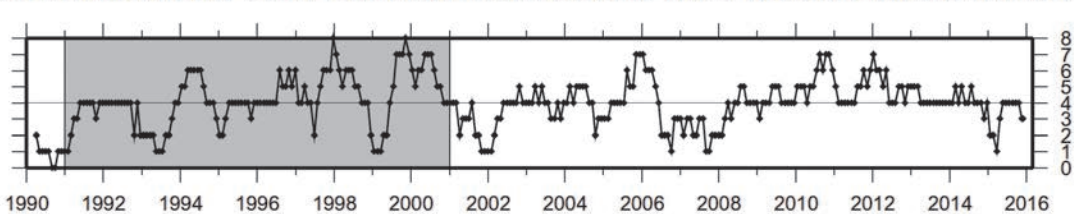
図3 東海地域の地震活動指数の推移
