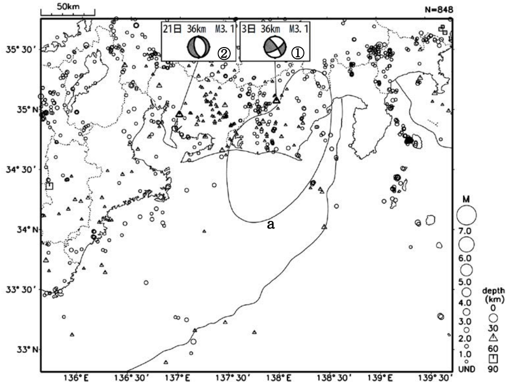
図1 震央分布図（2014年10月1日～31日：深さ0～90km、Mすべて。図中の領域aは東海地震の想定震源域。）
