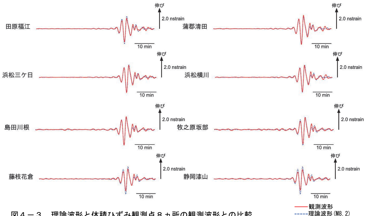
図 4-3 理論波形と体積ひずみ観測点 8 カ所の観測波形との比較
