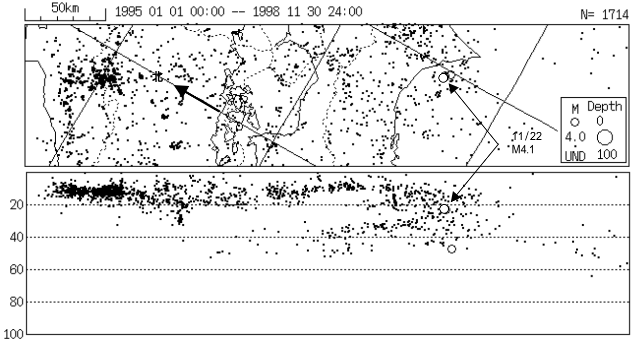
図6-1 土佐湾の地震活動（表示期間：1995年1月～1998年11月）
