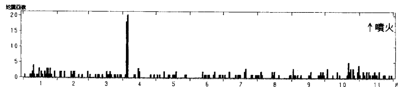
図 2 日別地震回数（1998年1月～11月）
