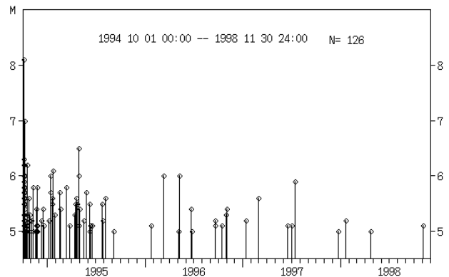
図 3 - 1 1994 年の北海道東方沖地震(M:8.1)の余震活動
