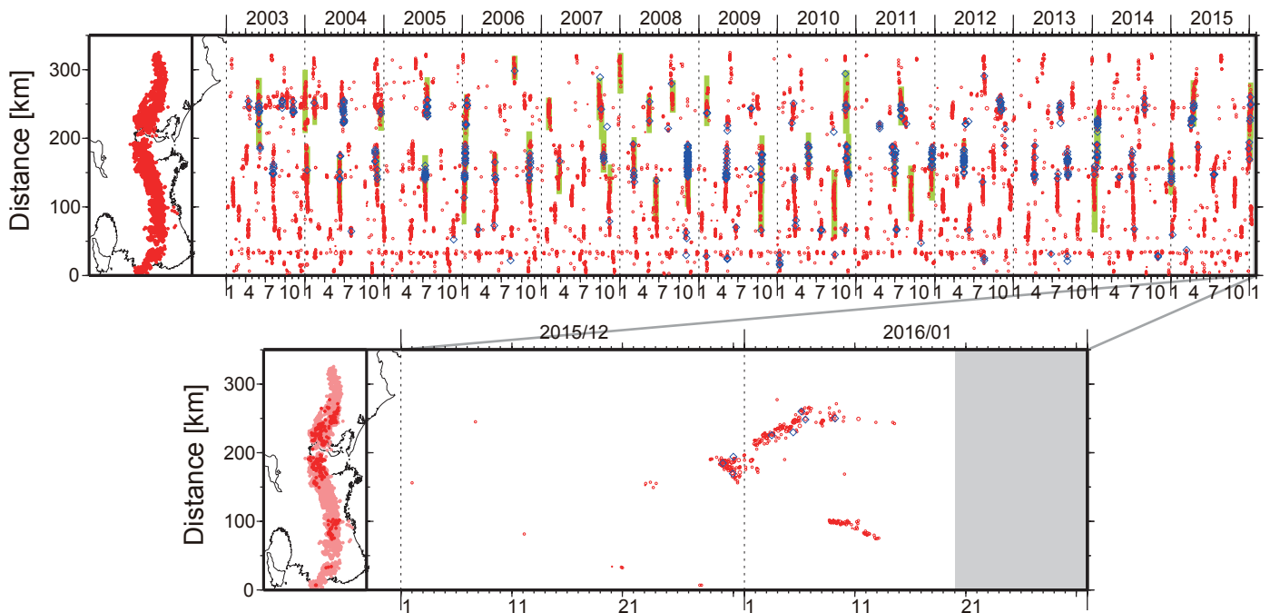
図 1. 紀伊半島・東海地域における 2003 年 1 月～2016 年 1 月 19 日までの深部低周波微動の時空間分布 (上図). 赤丸はエンベロップ相関・振幅ハイブリッド法 (Maeda and Obara, 2009) およびクラスタ処理 (Obara et al., 2010) によって 1 時間毎に自動処理された微動分布の重心である. 青菱形は周期 20 秒に卓越する超低周波地震 (Ito et al., 2007) である. 黄緑色の太線はこれまでに検出された短期的スロースリップイベント (SSE) を示す. 下図は 2015 年 12 月～2016 年 1 月の拡大図である. 12 月 28 日～1 月 14 日頃に三重県北部から愛知県で微動活動がみられた. この活動は, 12 月 31 日頃まで南西方向に活動域が拡大したのち, 1 月 1 日頃からは伊勢湾を挟んだ愛知県西部の領域で活動が開始した. その後, 東方向への活動域の移動がみられ, 愛知県東部まで達した. 活動は 10 日頃より弱まりつつ 14 日頃まで継続した. この活動に際して, 傾斜変動から短期的 SSE の断層モデルも推定されている. 1 月 8 日～13 日頃には奈良県南部でやや活発な微動活動が発生し, 西方向への活動域の移動がみられた. 12 月 20～21 日頃には, 和歌山県中部でごく小規模な活動がみられた. 12 月 23～24 日頃には, 三重県北部で小規模な活動がみられた.
