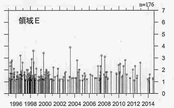
M-T図
