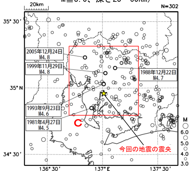
震央分布図
