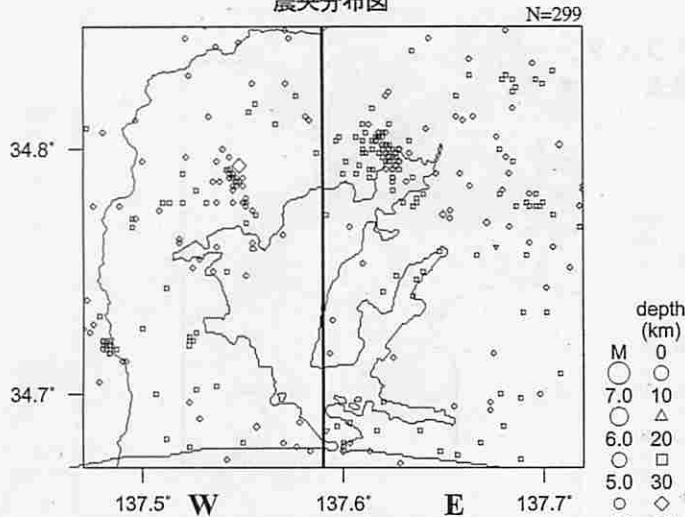
震央分布図
