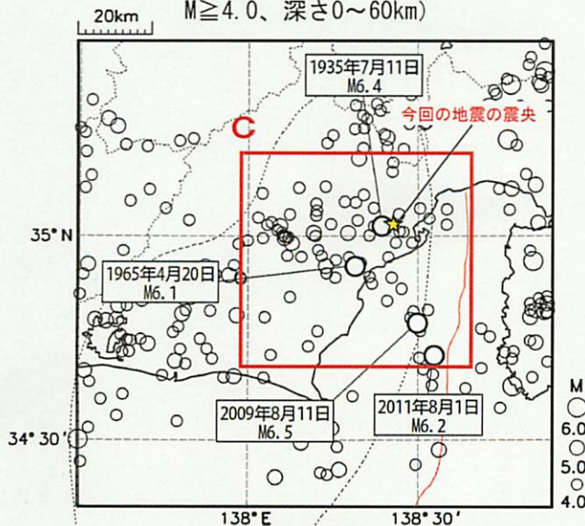
震央分布図
