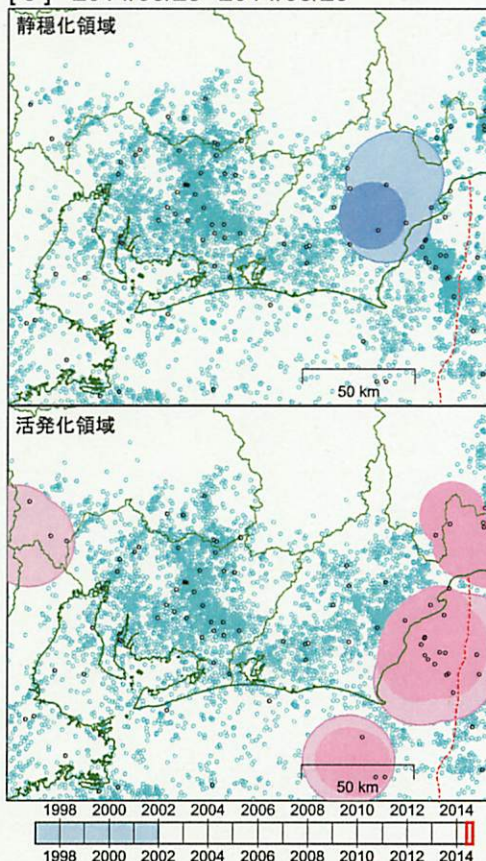
[ 3 ] 2014/05/23--2014/08/20
