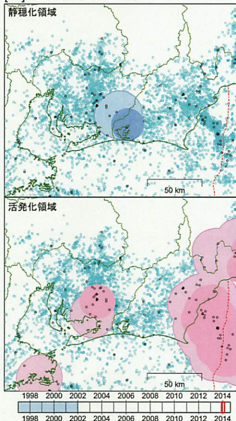
[ 1 ] 2013/11/24--2014/02/21
