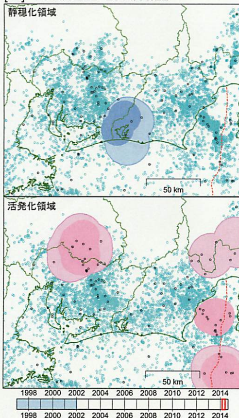
[ 2 ] 2014/02/22--2014/05/22
