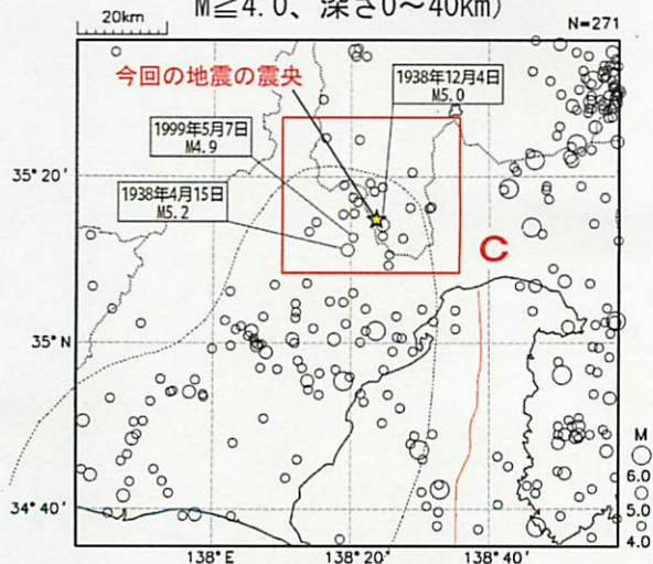
震央分布図 (1923年1月1日～2014年8月20日、 M \geq 4.0 、深さ0～40km)
