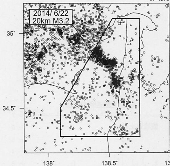
震央分布図
