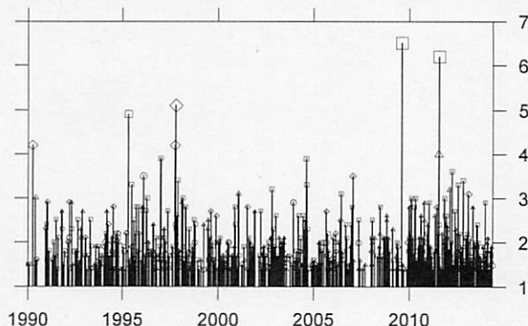
M-T図
