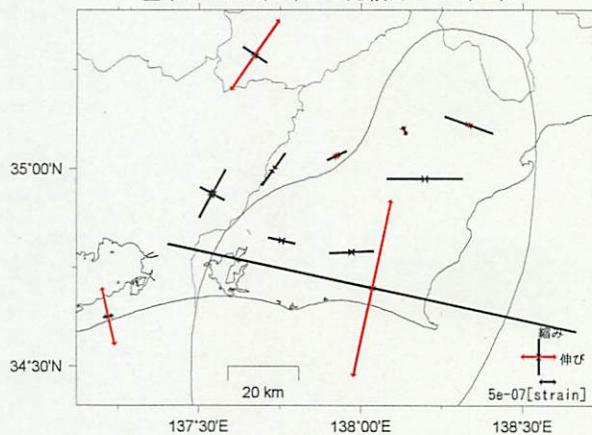
基準日：2013/08/03 比較日：2013/11/01
