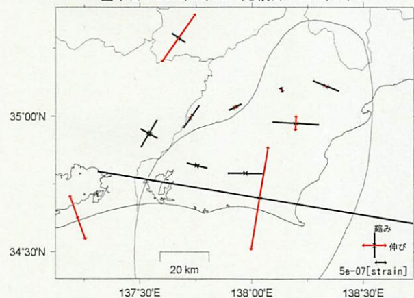
基準日：2013/11/03 比較日：2014/02/01
