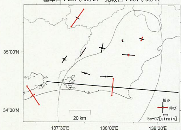
基準日：2014/02/21 比較日：2014/05/22
