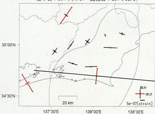
基準日：2014/01/31 比較日：2014/05/01
