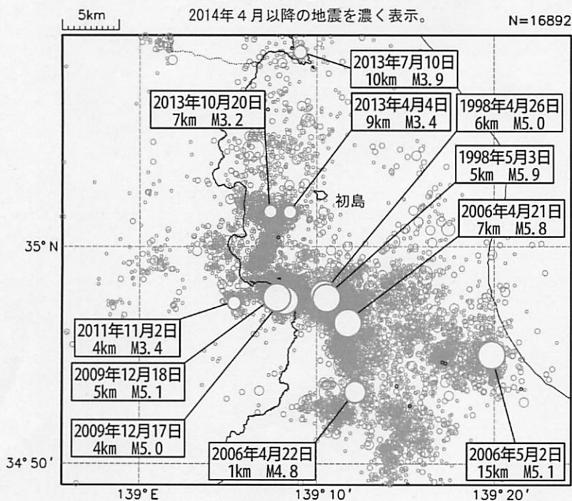
震央分布図（1997年10月1日～2014年5月21日、 M \geq 0.5 、深さ0～20km）
