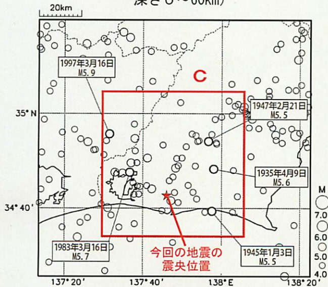
震央分布図
