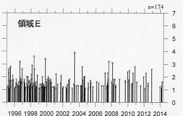
M-T図
