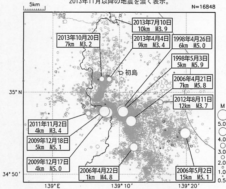
震央分布図（1997年10月1日～2013年12月18日、 M \geq 0.5 、深さ0～20km）
