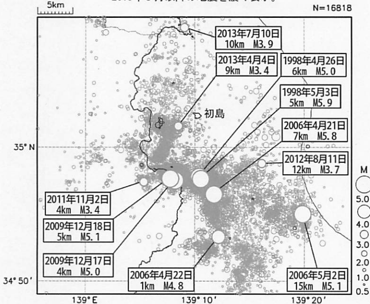
震央分布図（1997年10月1日～2013年10月16日、 M \geq 0.5 、深さ0～20km）
