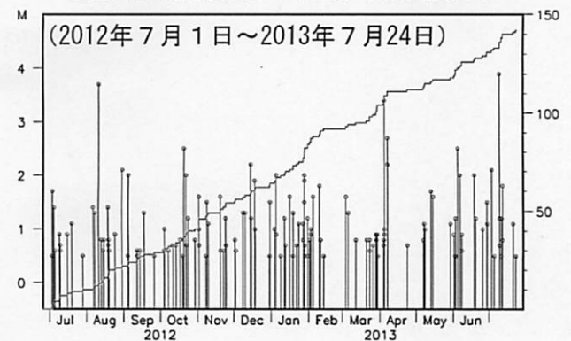
左図内の地震のM-T図、回数積算図
