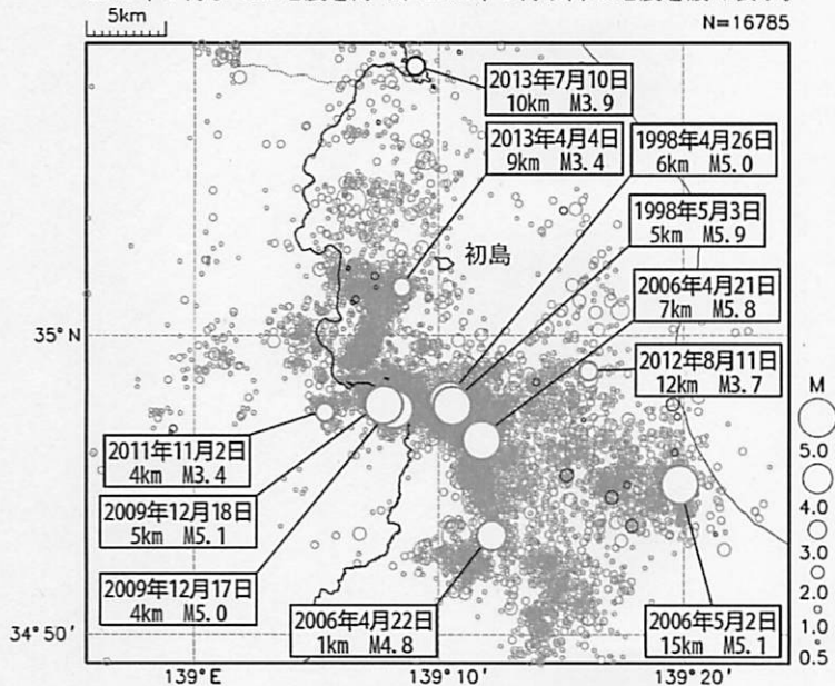
震央分布図 (1997年10月1日～2013年7月24日、 M \geq 0.5、深さ 0～20km)
