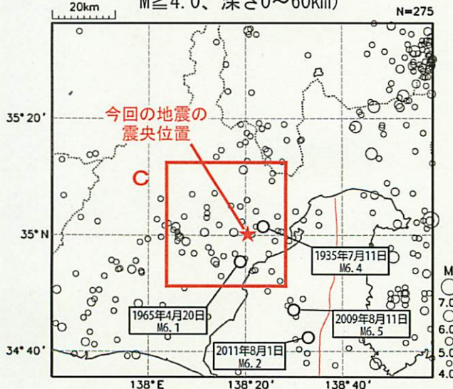
震央分布図 (1923年1月1日～2013年7月24日、 M \geq 4.0 、深さ0～60km)
