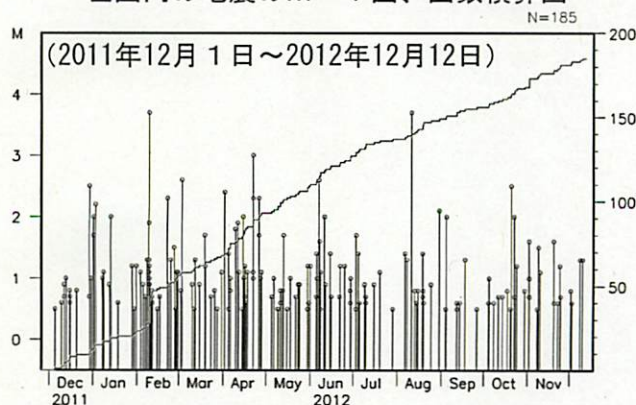
左図内の地震のM-T図、回数積算図
