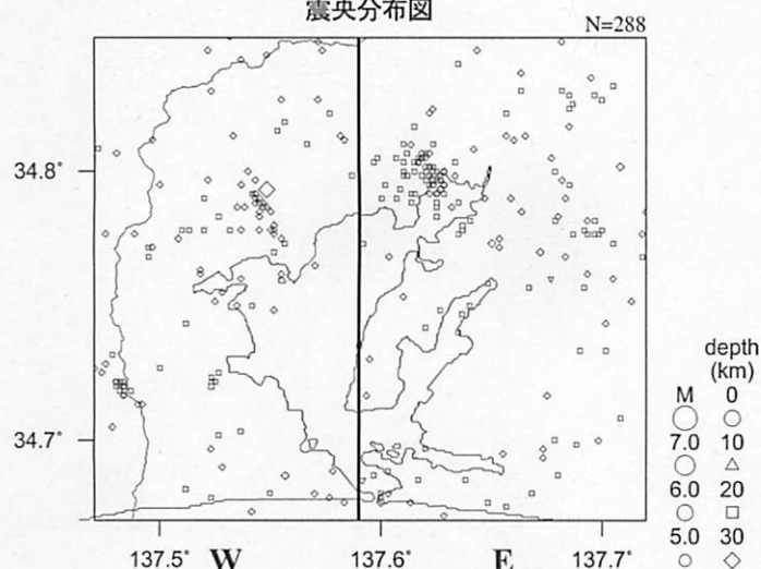
震央分布図
