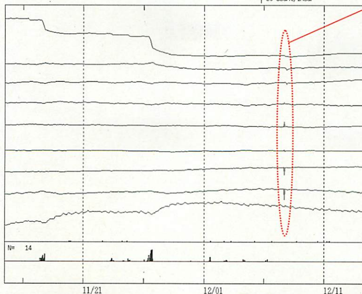
東伊豆地域の体積ひずみ計・傾斜計の記録 （2012年11月14日11時～12月14日11時）
