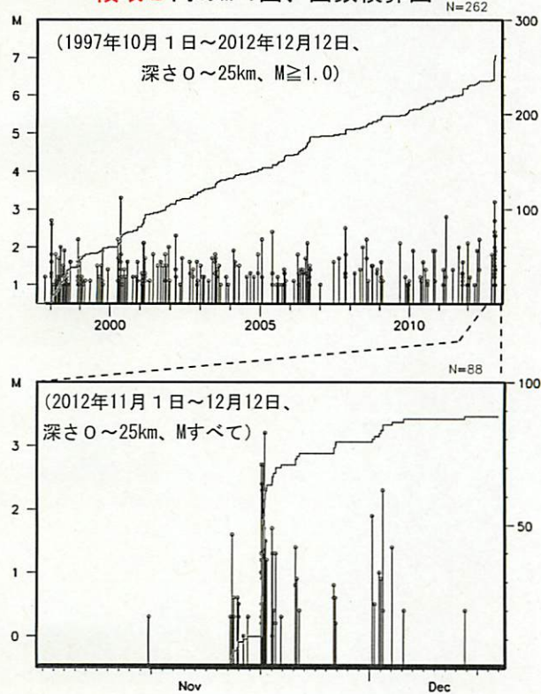
領域c内のM-T図、回数積算図
