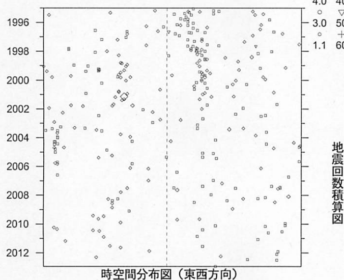
M-T 図
