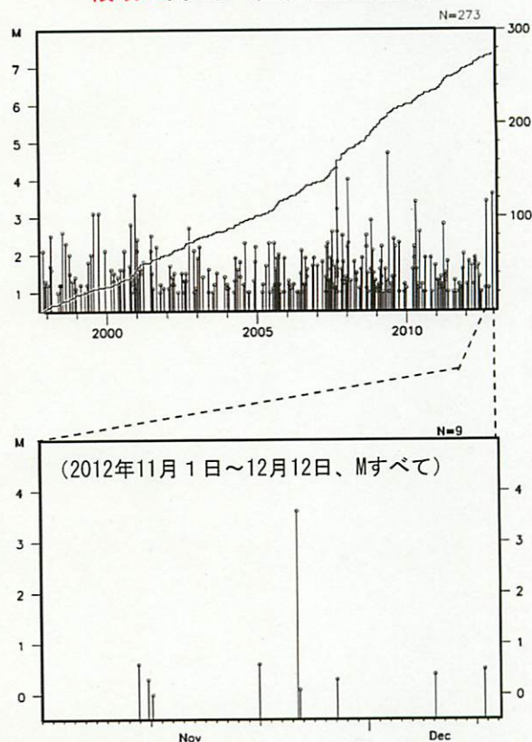
領域b内のM-T図、回数積算図
