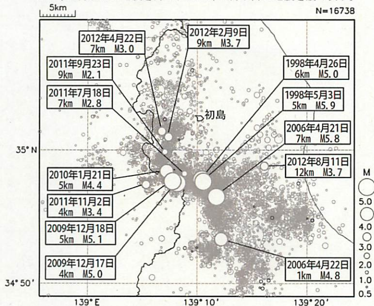
震央分布図（1997年10月1日～2012年12月12日、 M \geq 0.5 、深さ0～20km）
