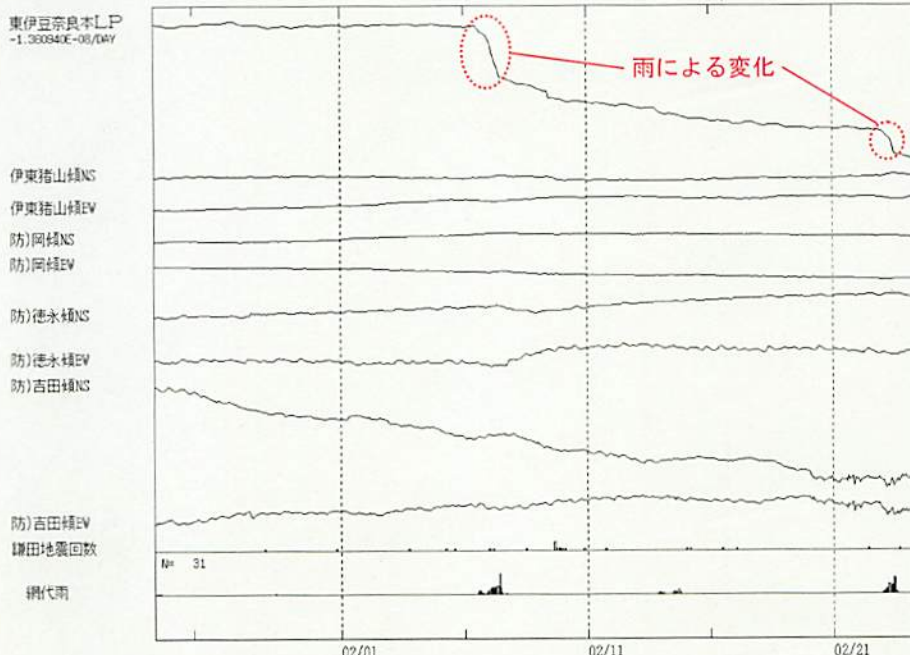
東伊豆地域の体積ひずみ計・傾斜計の記録 （2012年1月24日10時～2月24日10時）
