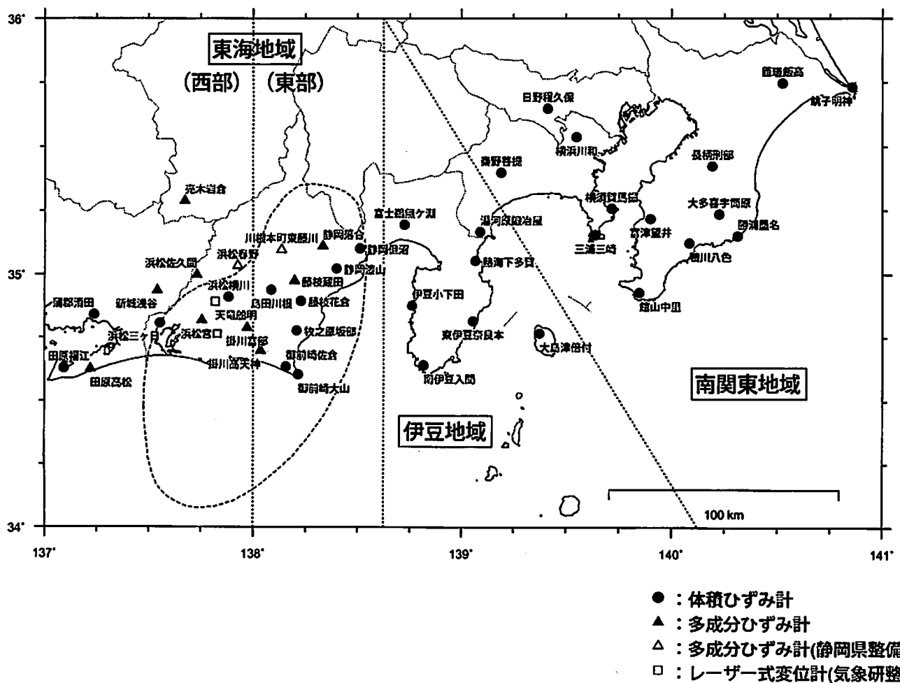
ひずみ計の配置図
