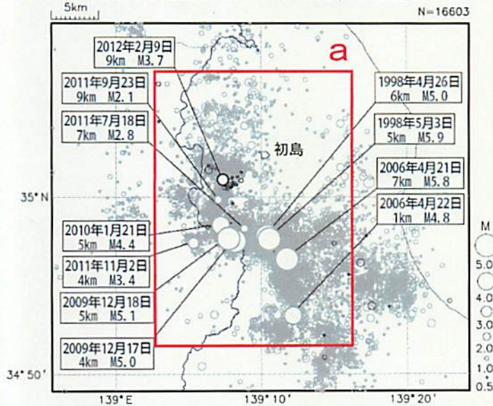
震央分布図（1997年10月1日～2012年2月22日、 M \geq 0.5 、深さ0～20km）
