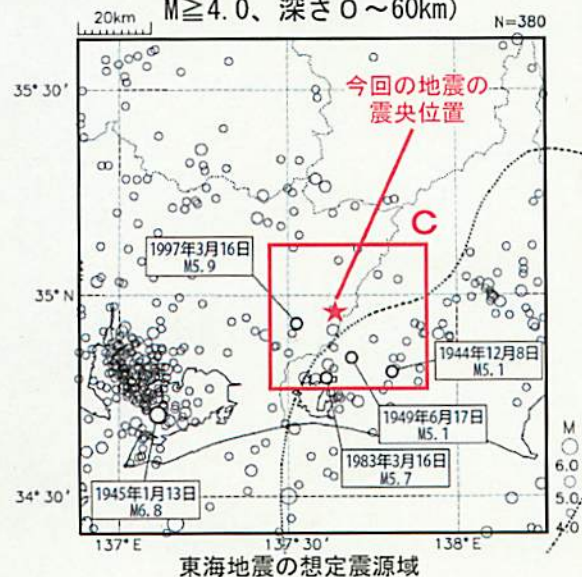
震央分布図（1923年8月1日～2012年2月19日、 M \geq 4.0 、深さ0～60km）
