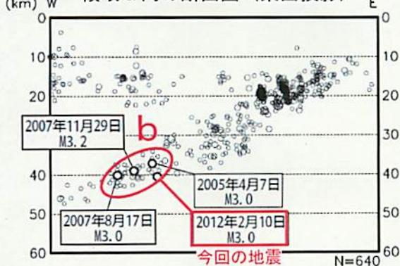
領域a内の断面図（東西投影）
