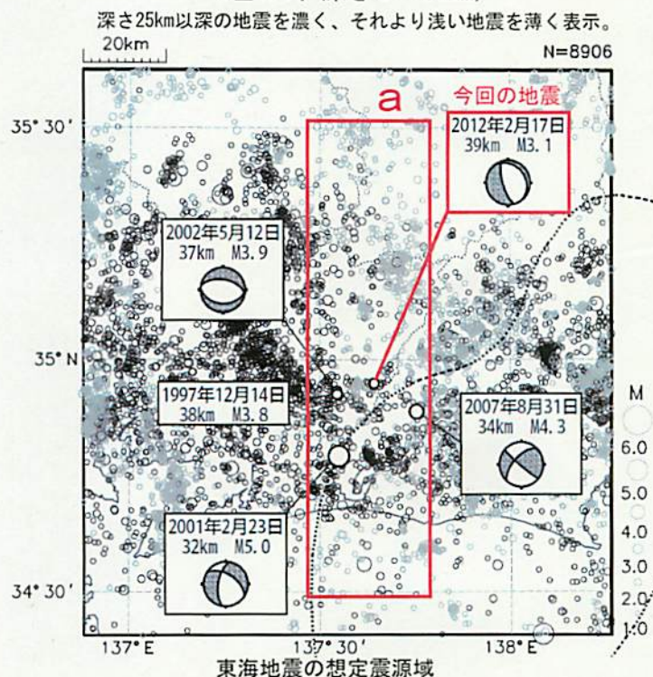
震央分布図（1997年10月1日～2012年2月19日、 M \geq 1.0 、深さ0～60km）
