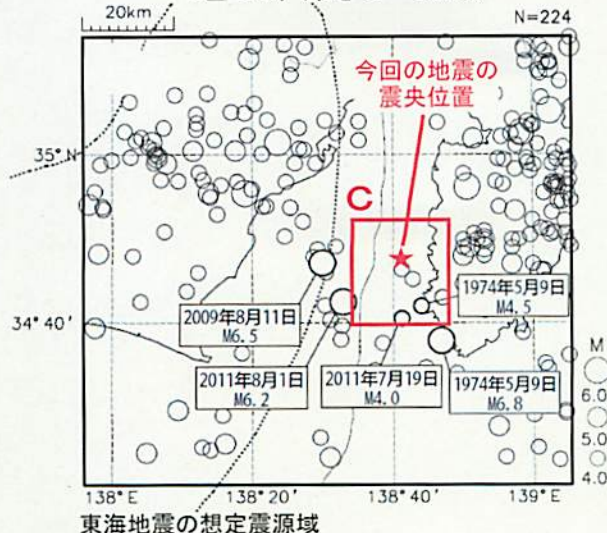
震央分布図（1923年8月1日～2012年2月19日、 M \geq 4.0 、深さ0～50km）
