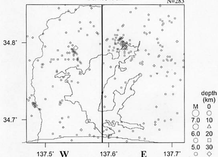
震央分布図
