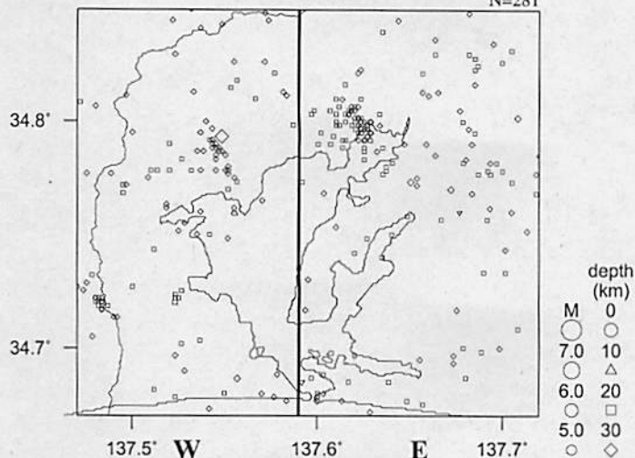
震央分布図
