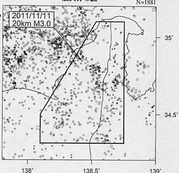
震央分布図
