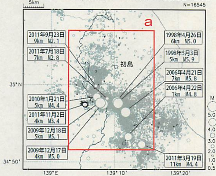
震央分布図（1997年10月1日～2011年11月16日、 M \geq 0.5 、深さ0～20km）
