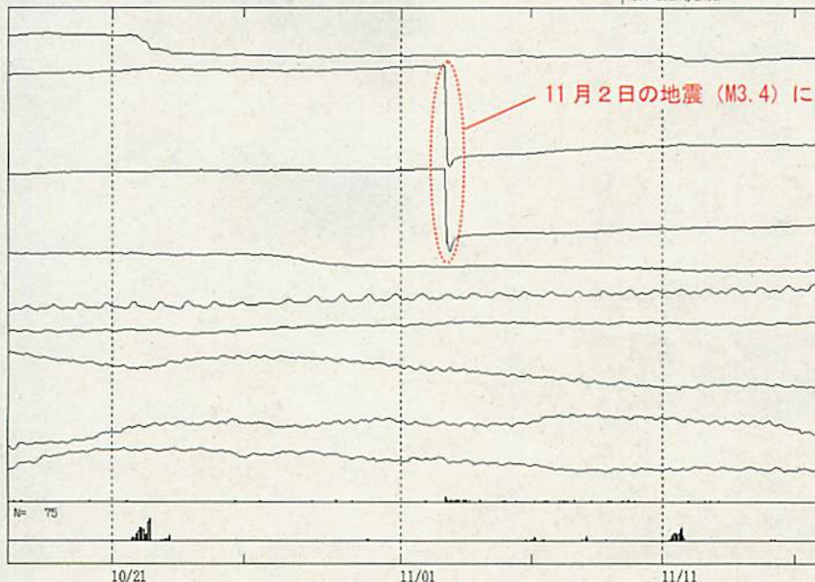
東伊豆地域の体積ひずみ計・傾斜計の記録 （2011年10月17日～11月16日）
