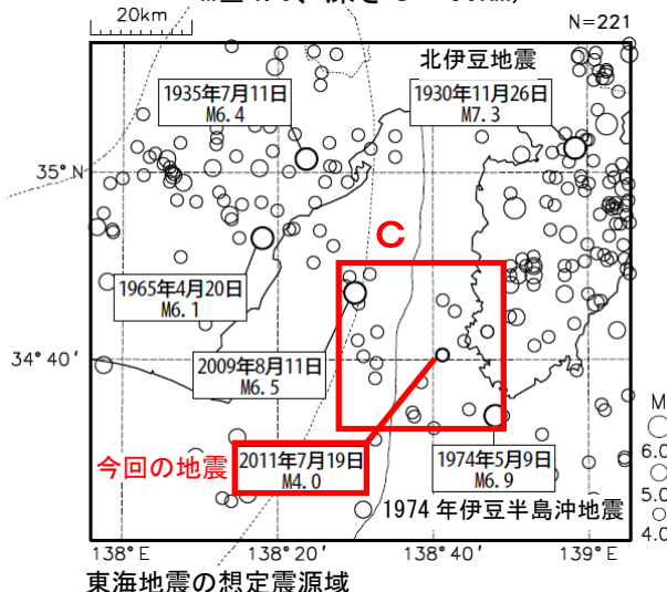
震央分布図（1923年8月1日～2011年7月20日、 M \geq 4.0 、深さ0～50km）
