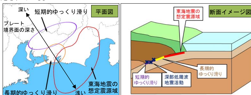
東海地震想定震源域、並びに長期的ゆっくり滑り及び短期的ゆっくり滑りの発生領域
