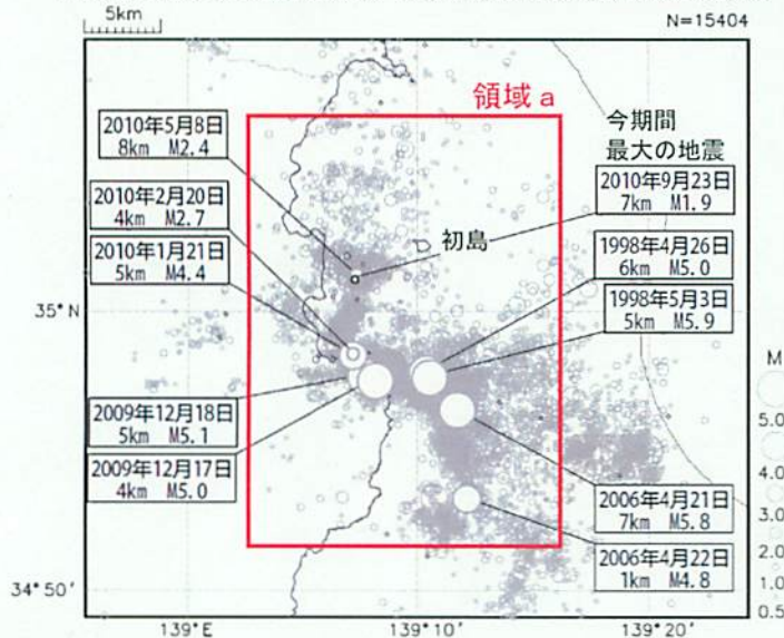
震央分布図（1997年10月1日～2010年9月23日、 M \geq 0.5 、深さ0～20km）
