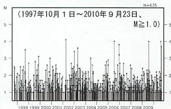
今回の地震の震央から半径3kmの範囲内で発生した地震の活動経過図
