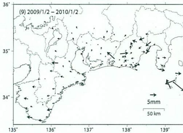
【水平変動】
