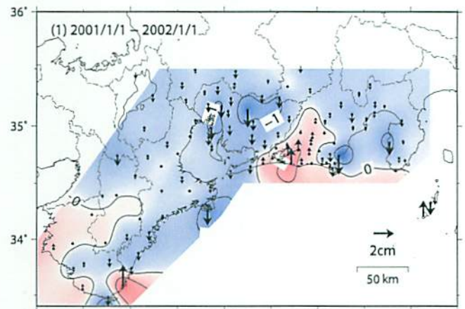
【上下変動】
