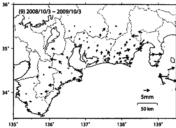
【水平変動】
