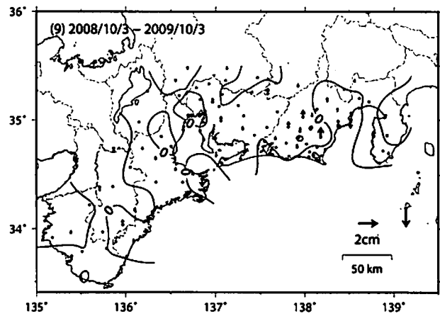
【上下変動】
