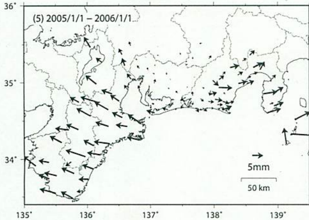
【水平変動】
