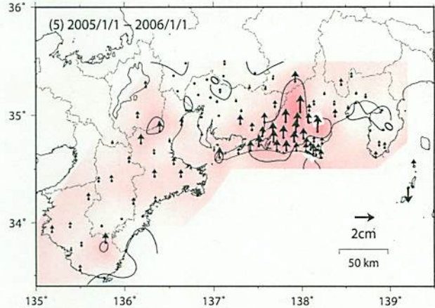
【上下変動】
