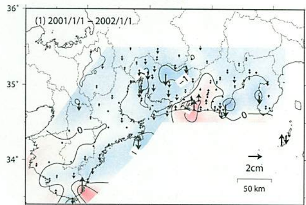
【上下変動】
