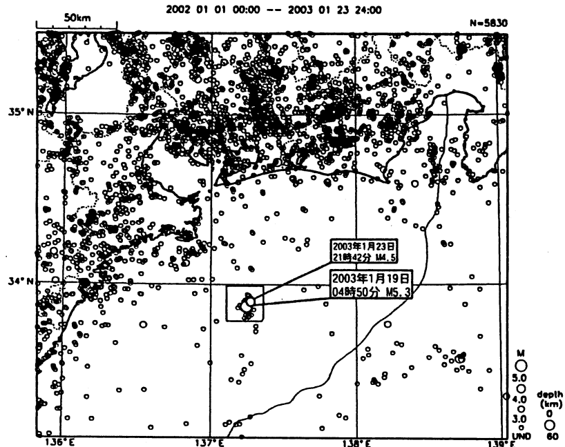
矩形内の地震活動経過図 (規模別)
