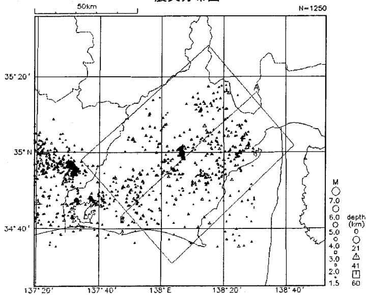
(2) M \geq 1.5 震央分布図
