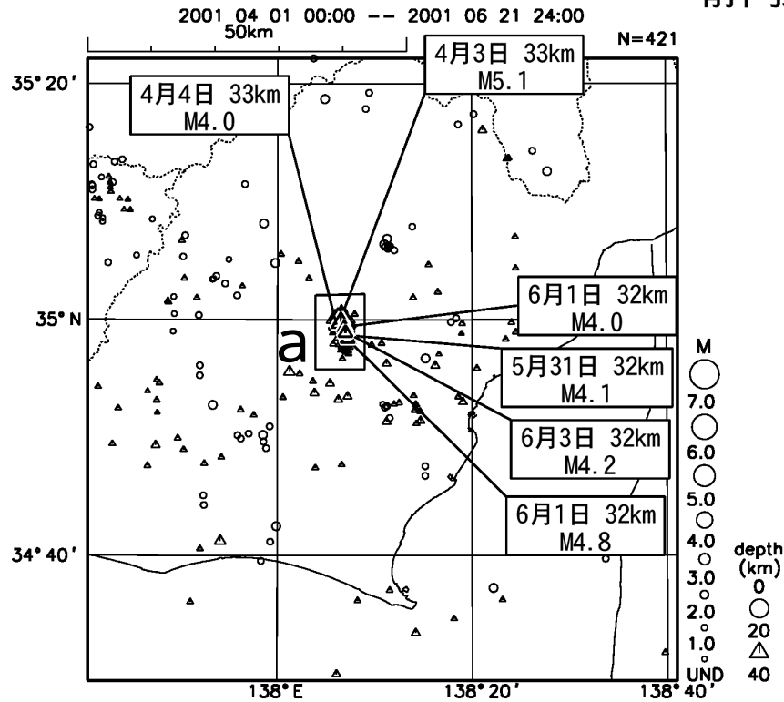
領域aの地震活動経過図(規模)
